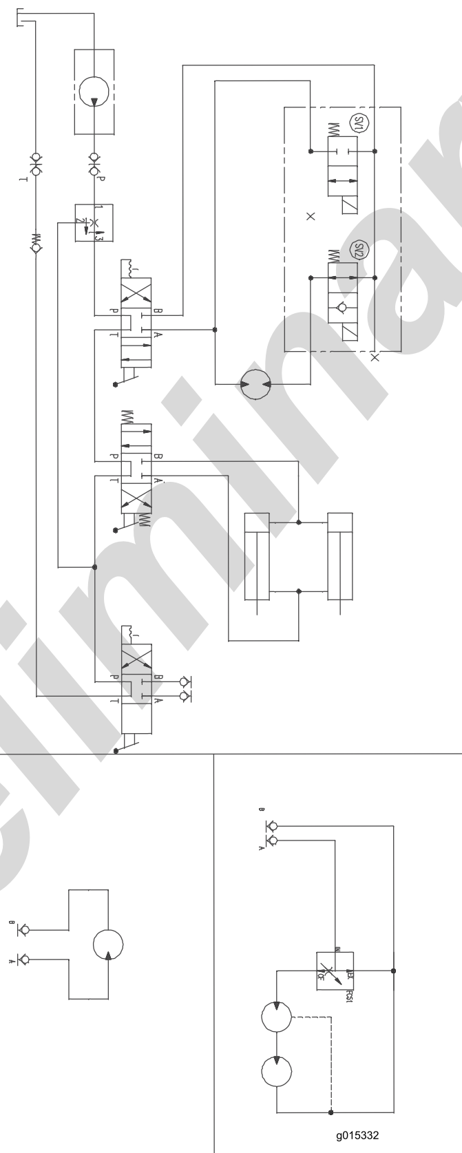
Schemat hydrauliczny – modele SH (Rev. -)
