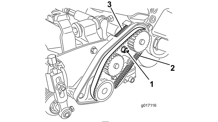
1. 轴承座安装螺母 3. 压缩弹簧 2. 滚刀传动皮带
