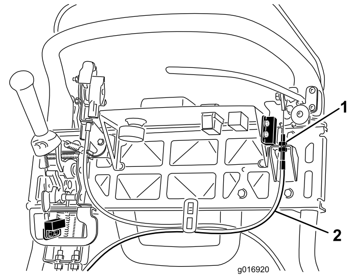
1. 锁紧螺母 2. 刹车拉线
