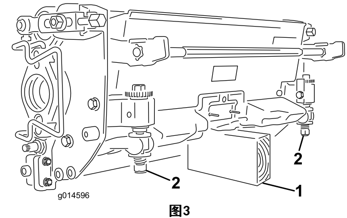
1. 支撑块（未提供） 2. 底刀调节螺丝（2）
