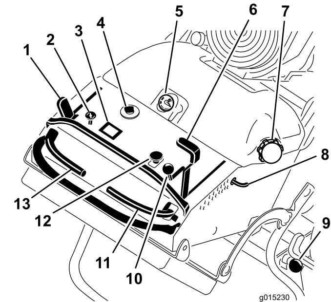
Figura 6 Máquinas de 48 y 52 pulgadas
