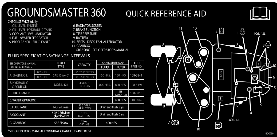
Figuur 28 Onderhoudsschema
