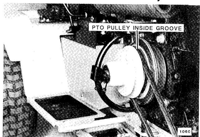
FIG. 9. Mower PTO Pulley
