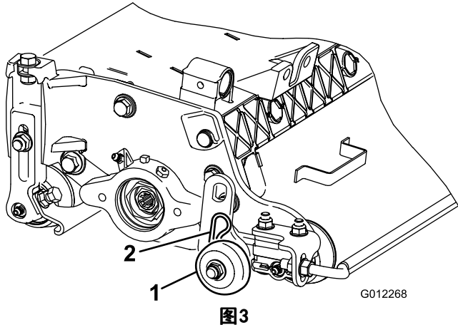
1. 行走滚筒总成 2. 开口销
