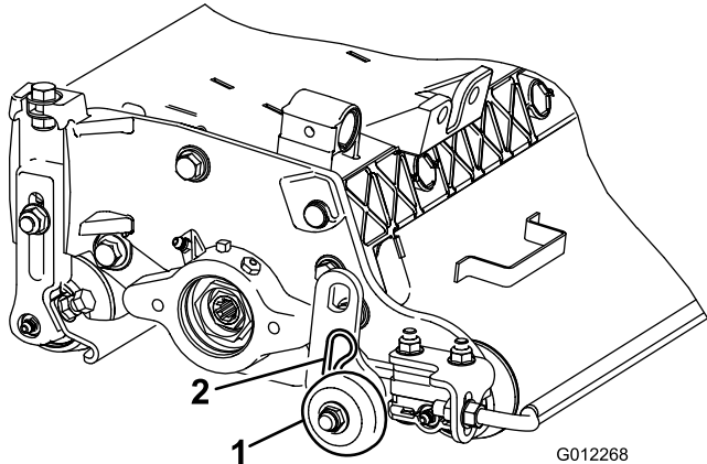
1. 行走滚筒总成 2. 开口销
