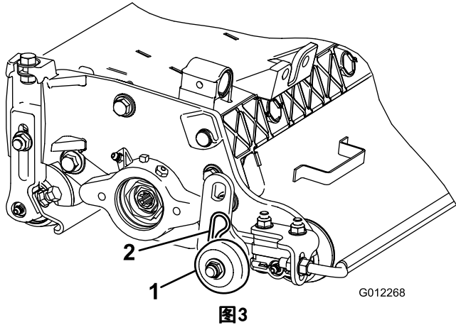
1. 行走滚筒总成 2. 开口销
