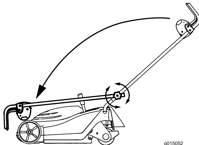
Figure 21 Modèle 21141 montré
