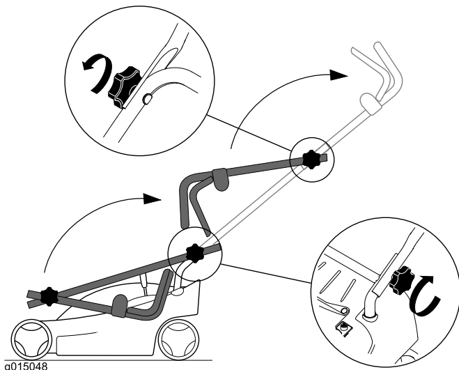
Figure 1 Modèle 21136
