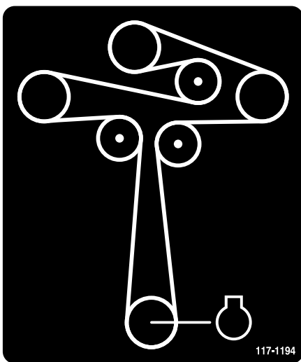
Figure 4 Acheminement de la courroie
