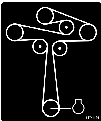
Figuur 4 Geleiding van drijfriem
