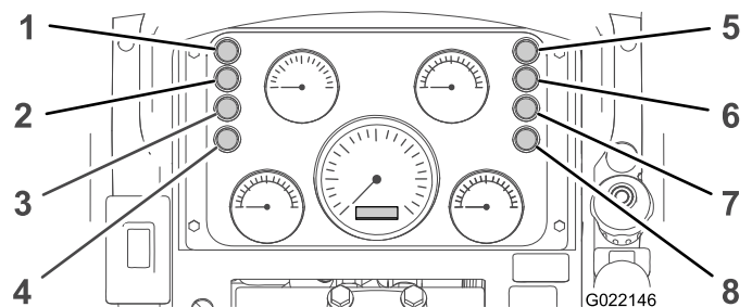
Bild 8 Armaturenbrettlampen
