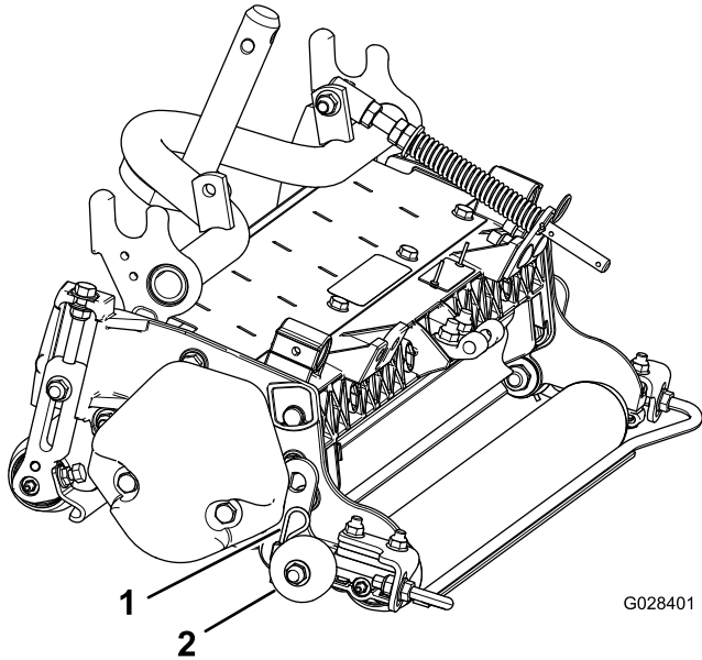
1. 开口销 2. 行走滚筒总成
