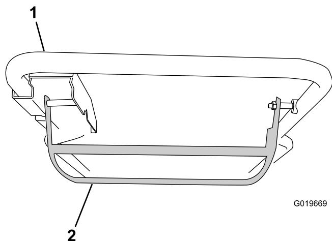
Figur 13 Styrstång
