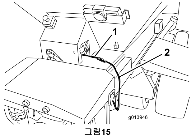
1. 파워 하니스
