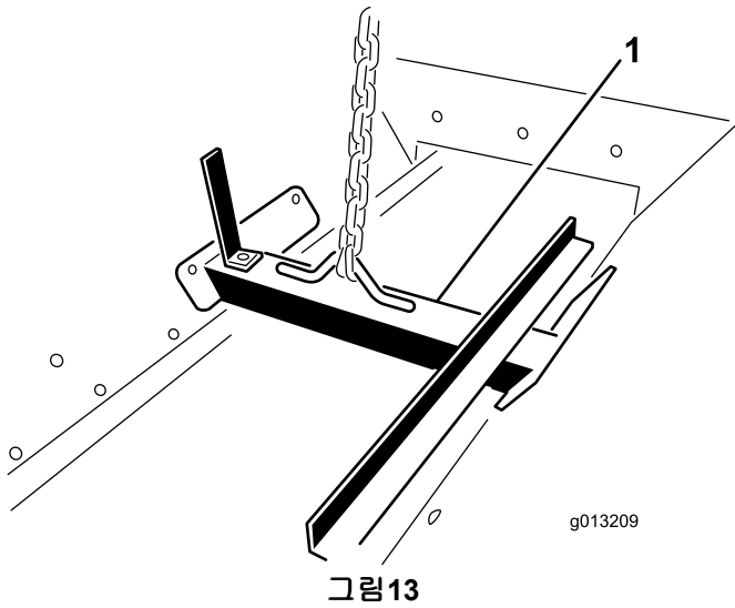
1. 리프팅 브래킷
