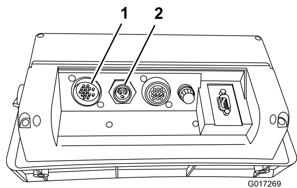
图3 控制台电脑的后部
