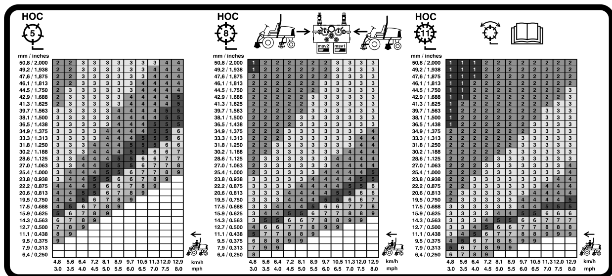
図 34 7 インチ 177.8mm リールの速度表
