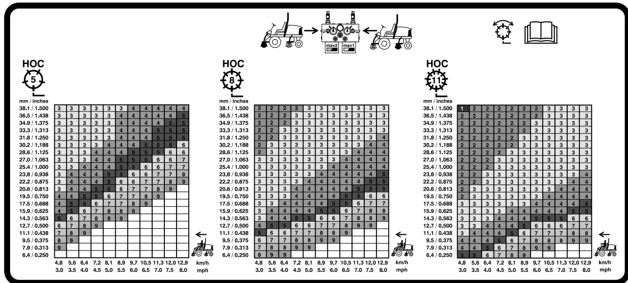
図 33 5 インチ127mmリールの速度表
