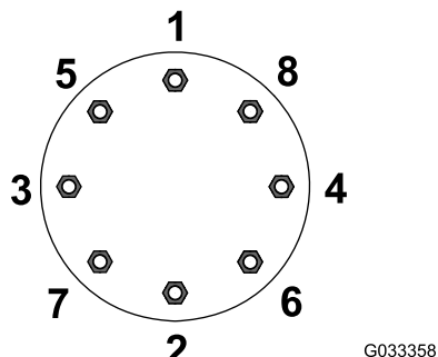
Figura 10 Ruote anteriori
