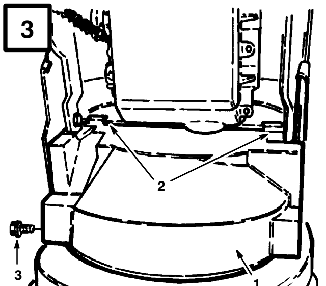
1. Nederste remdeksel (vist fra bunnen) 2. Monteringsflenser 3. Flenshodeskruer
