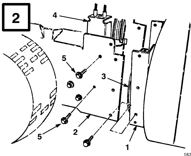
1. Spiralbladhus 2. Motorramme 3. Remskive for viftehjul 4. Lederull -enhet 5. Monteringsskruer (2)
