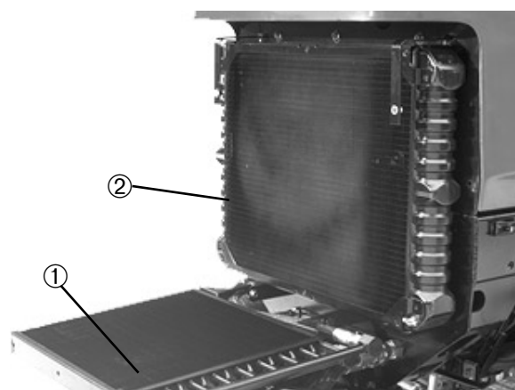
Fig. 40 1. Oliekoøler 2. Køler
