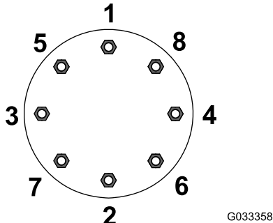
Bild 10 Vorderräder
