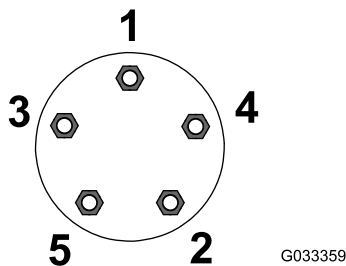
Bild 11 Hinterräder
