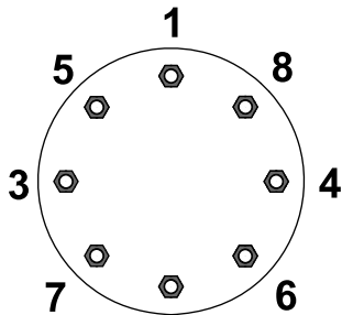
Figur 10 Framhjul
